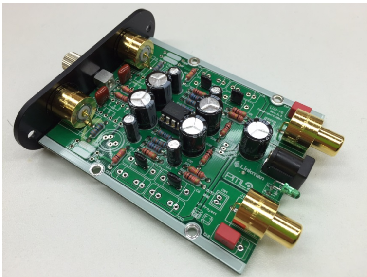
LA-RCAJ-S (4個) を取り付けした LV2-PE
