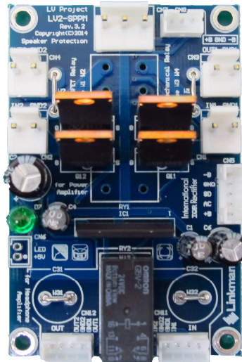
パワーアンプ (FET), ヘッドフォンアンプ (リレー)
